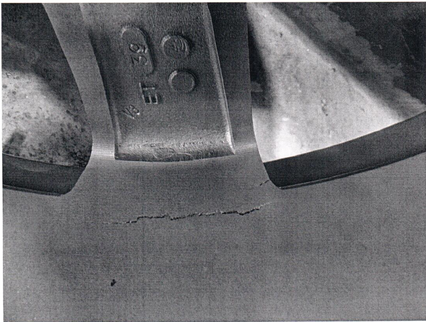
Рисунок 1а – Трещина в соединении спицы с ободом.
