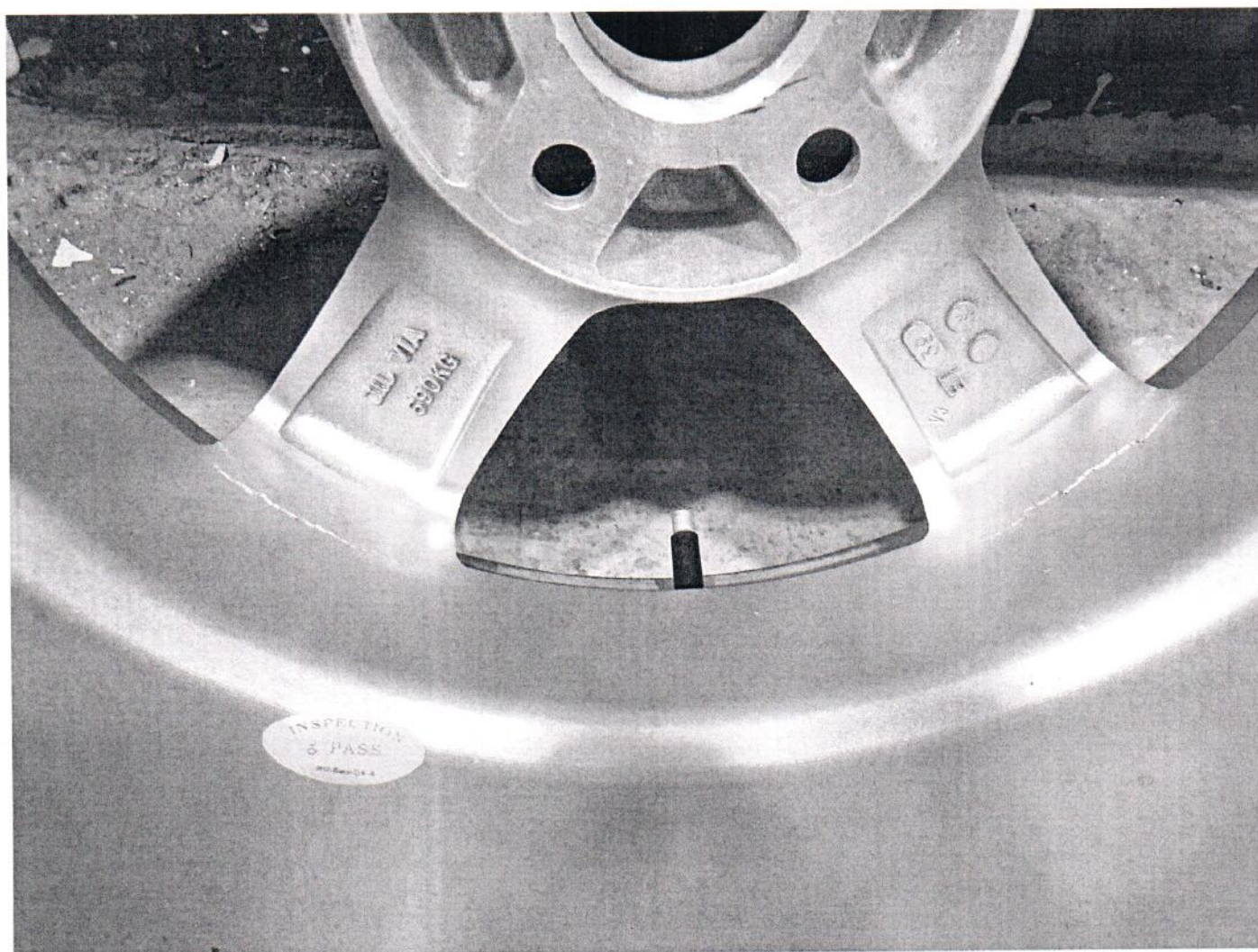
Рисунок 1 – Трещины в соединении спиц с ободом.
