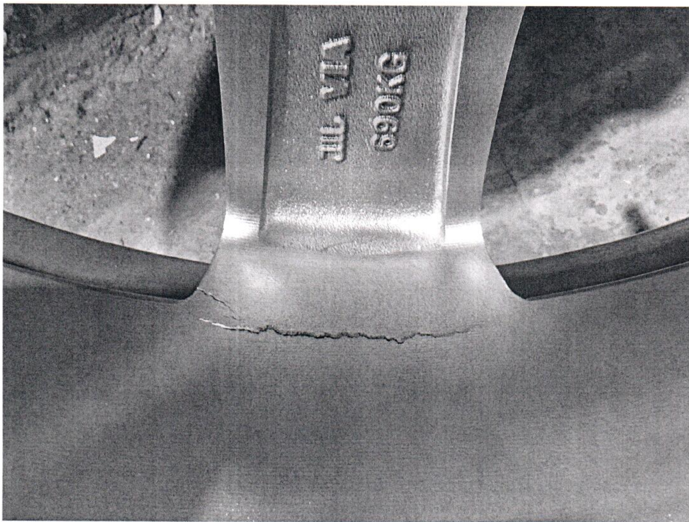
Рисунок 1в – Трещина в соединении спицы с ободом.
