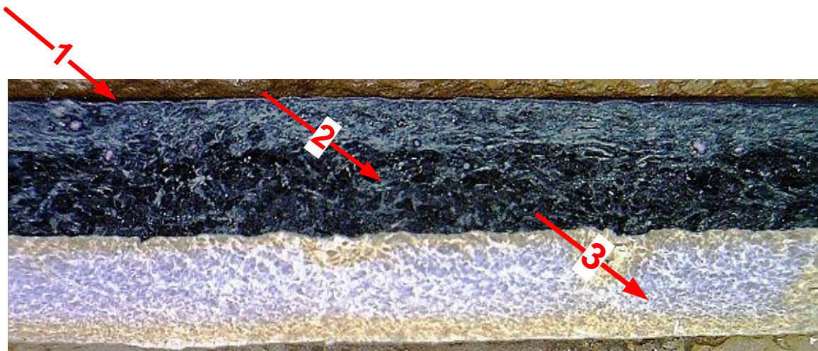
Рис. 3 Поперечный срез материалов (1) обуви - 1 – пленочное покрытие, 2 -кожевенные волокна верха обуви, 3 – кожевенные волокна подкладки
