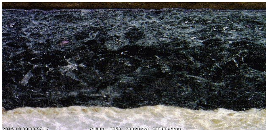
Рис. 4 Кожевенные волокна верха (1) обуви под пленочным поверхностным покрытием
